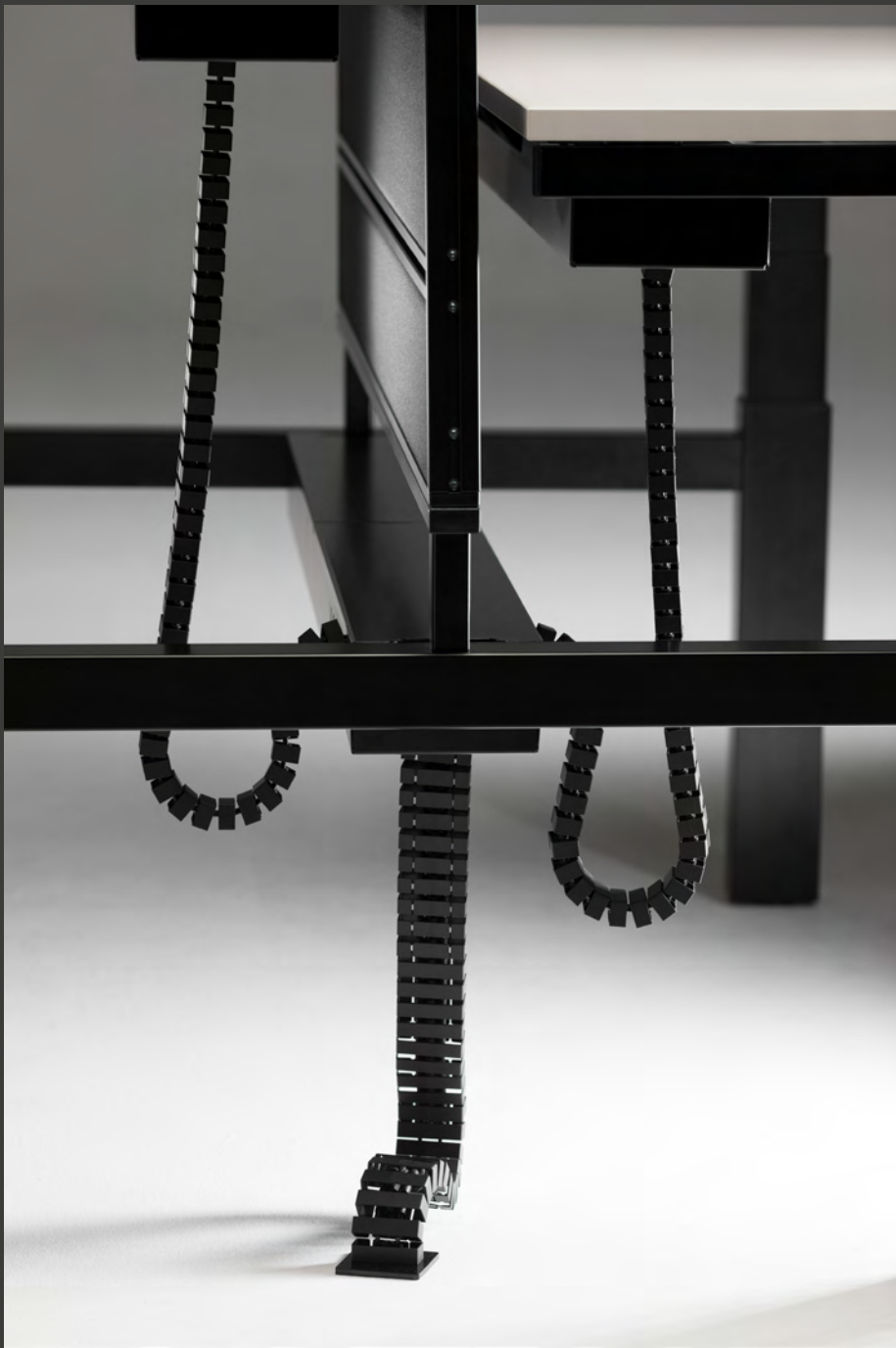
Vertikale Kabelkanäle, flexibel und modular, für Workbench-Arbeitsplätze, verbunden mit dem gemeinsamen horizontalen Kabelkanal | Goulotte verticale, flexible et modulaire, pour benches, attachée à la goulotte horizontale partagée
